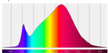
Spectra
